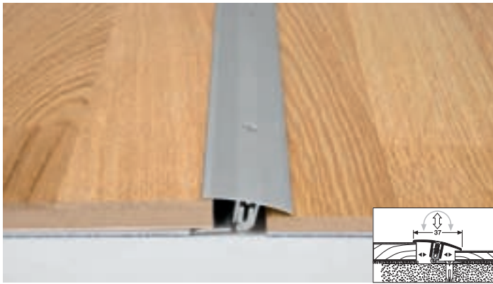
Typ 888 Universal-Übergangsprofil »Flex« | 7 bis 17 mm
