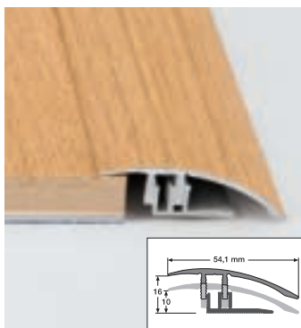
Typ 586 E Klipp-Anpassungsprofil 10 bis 16 mm
