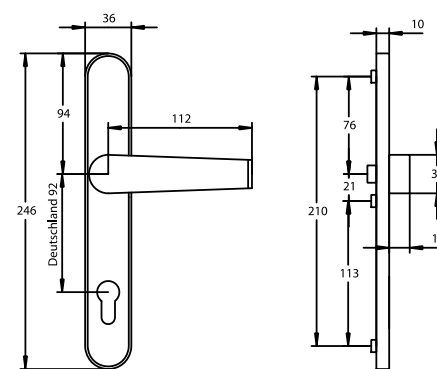
Außenhalbgarnitur mit Flachdrücker
