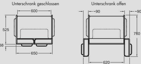
Handtuchhalter, Boden/Zwischenboden optional
