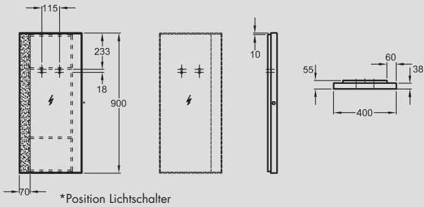
14 Lichtspiegelement, links/rechts, Rahmen verchromt, Leuchte T5 FH, 21 W, 220-240 V, 50-60 Hz, Anti-Beschlag, Lichtschalter, IP 44, Schutzklasse 2, 400 x 900 x 55 mm, Modell-Nr. 816540.
