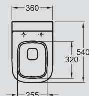
15 Tiefspül-WC, 6 l, wandhängend, 360 x 540 mm, Modell-Nr. 201400. WC-Sitz, Modell-Nr. 575400. WC-Sitz mit Absenkautomatik, Modell-Nr. 575410.
