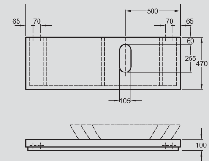
7 Waschtischplatte, Siphonausschnitt rechts, umlaufende Blende in Chrom-Optik, inkl. Montagekonsolen, 1400 x 100 x 470 mm, Modell-Nr. 816641 Weiß Hochglanz. Kombinierbar mit Aufsatzwaschtisch, Ablagefläche rechts, Waschtischen 600 · 800 · 1000 mm, Waschtischunterschrank 600 · 1400 mm, Handtuchhalter 430 · 760 mm und Kosmetik-Modulen.
