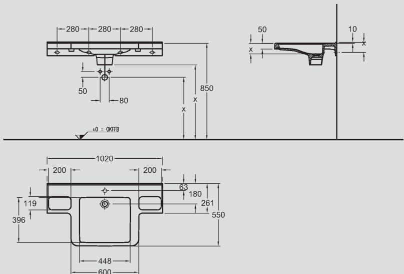
2 Waschtisch aus Varicor®, ohne Überlauf, seitliche Ablageflächen und zwei Multifunktionslöcher, 1020 x 550 mm, Modell-Nr. 470025.
