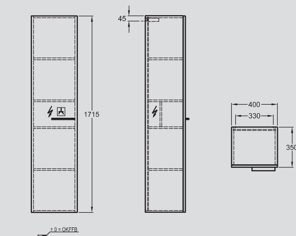
13 Hochschrank, 1 Tür, Anschlag rechts/links, 1 Griff, verchromt, 4 Einlegeböden, mit Spiegel auf der Innentür und Lichtleiste, inkl. Transformator 230 V/12 V, 400 x 1715 x 350 mm, Modell-Nr. 816002 Weiß Hochglanz.
