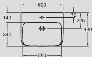
1 Waschtisch mit Ablaufkappe Weiß/Chrom, 600 x 480 mm, Modell-Nr. 125460. Kombinierbar mit Halbsäule, Modell-Nr. 291410 und Waschtischunterschränken 495 mm. Auch mit Ab- und Überlaufsystem Clou erhältlich.
