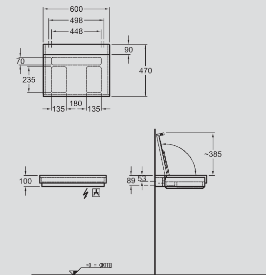
9 Kosmetik-Modul, aufklappbar, mit Spiegel und Licht, umlaufende Blende in Chrom-Optik, 600 x 100 x 470 mm, Modell-Nr. 816352 Weiß Hochglanz. Kombinierbar mit allen Waschtischplatten.
