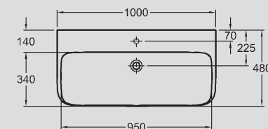
4 Waschtisch mit Ablaufkappe Weiß/Chrom, 1000 x 480 mm, Modell-Nr. 125400. Kombinierbar mit Halbsäule, Modell-Nr. 291410 und Waschtischunterschränken 880 mm. Auch mit Ab- und Überlaufsystem Clou erhältlich.
