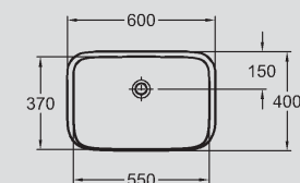
6 Einbauwaschtisch mit Ablaufkappe Weiß/Chrom, 600 x 400 mm, Modell-Nr. 245460. Kombinierbar mit Waschtischunterschränken 1150 mm.
