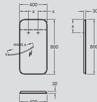
17 Lichtspiegelement, 400 x 800 x 30 mm, Modell-Nr. 814340.
