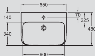
2 Waschtisch mit Ablaufkappe Weiß/Chrom, 650 x 480 mm, Modell-Nr. 125465. Kombinierbar mit Halbsäule, Modell-Nr. 291410 und Waschtischunterschränken 540 mm. Auch mit Ab- und Überlaufsystem Clou erhältlich.
