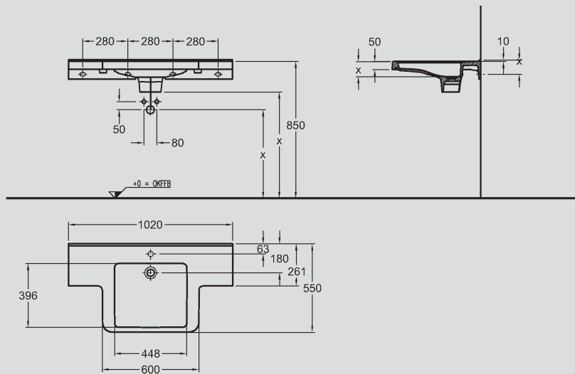
1 Waschtisch aus Varicor®, ohne Überlauf, seitliche Ablageflächen, 1020 x 550 mm, Modell-Nr. 470020.
