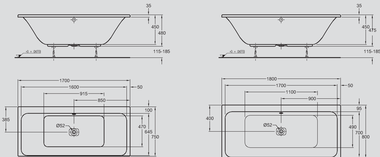
21 Badewanne, Bohrung für Überlauf an Wandseite, Tiefe 450 mm. 1700 x 750 mm, Modell-Nr. 650570. 1800 x 800 mm, Modell-Nr. 650580.
