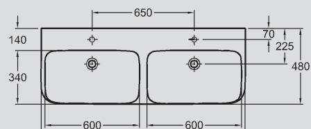
5 Doppelwaschtisch mit Ablaufkappen Weiß/Chrom, 1300 x 480 mm, Modell-Nr. 135430. Kombinierbar mit Halbsäule, Modell-Nr. 291410 und Waschtischunterschränken 1160 mm. Auch mit Ab- und Überlaufsystem Clou erhältlich.
