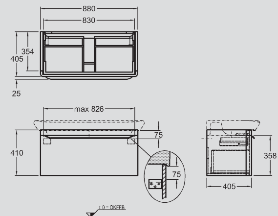
11 Waschtischunterschrank, 1 Auszug, Griff verchromt, 1 innenliegende Schublade, 880 x 410 x 405 mm. Modell-Nr. 814100 Weiß Hochglanz. Modell-Nr. 814101 Taupe Hochglanz. Kombinierbar mit Waschtisch 1000 mm.
