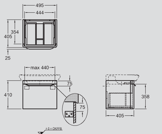
8 Waschtischunterschrank, 1 Auszug, Griff verchromt, 495 x 410 x 405 mm. Modell-Nr. 814060 Weiß Hochglanz. Modell-Nr. 814061 Taupe Hochglanz. Kombinierbar mit Waschtisch 600 mm.
