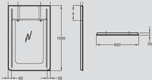
14 Lichtspiegelement, Power-LED 14 W, 220-240 V, 50-60 Hz, IP 44, Schutzklasse 2, 650 x 1000 mm, Modell-Nr. 808665.
