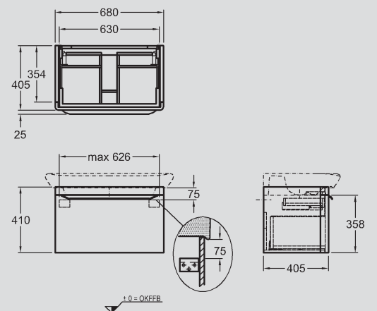
10 Waschtischunterschrank, 1 Auszug, Griff verchromt, 1 innenliegende Schublade, 680 x 410 x 405 mm. Modell-Nr. 814080 Weiß Hochglanz. Modell-Nr. 814081 Taupe Hochglanz. Kombinierbar mit Waschtisch 800 mm.
