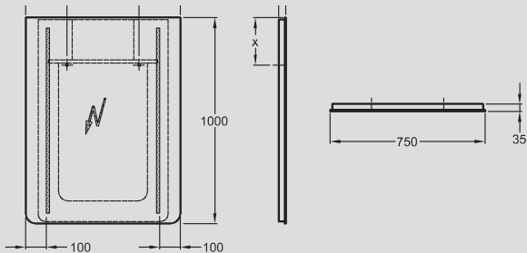
15 Lichtspiegelement, Power-LED 14 W, 220-240 V, 50-60 Hz, IP 44, Schutzklasse 2, 750 x 1000 mm, Modell-Nr. 808675.
