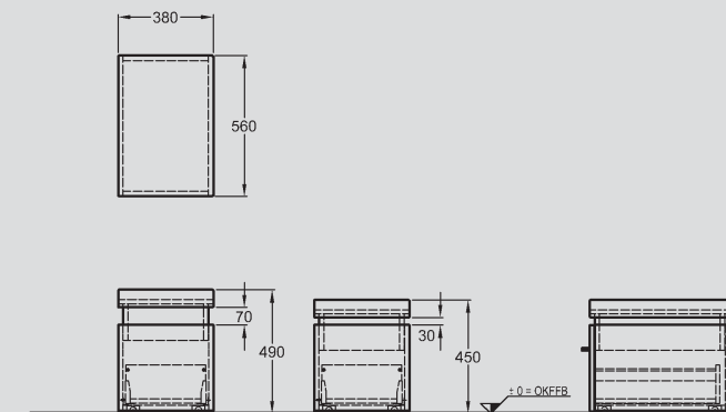
10 Hocker, in zwei Höhen verstellbar, mit Sitzkissen, 1 Auszug, 1 Griff, verchromt, mit Rollen, die bei Belastung stoppen, 380 x 450/490 x 560 mm, Modell-Nr. 816072 Weiß Hochglanz.
