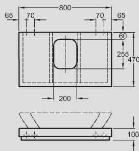
2 Waschtischplatte, Siphonausschnitt mittig, umlaufende Blende in Chrom-Optik, 800 x 100 x 470 mm, Modell-Nr. 816680 Weiß Hochglanz. Einzeln montierbar nur in Verbindung mit Montagekonsolen, Modell-Nr. 516200. Kombinierbar mit Waschtischen 600 · 800 mm, Waschtischunterschrank 800 mm, Handtuchhalter 430 mm (seitliche Montage) und Kosmetik-Modulen.
