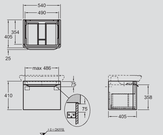
9 Waschtischunterschrank, 1 Auszug, Griff verchromt, 540 x 410 x 405 mm. Modell-Nr. 814065 Weiß Hochglanz. Modell-Nr. 814066 Taupe Hochglanz. Kombinierbar mit Waschtisch 650 mm.
