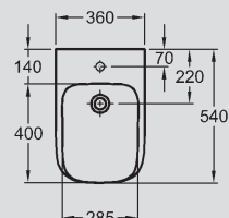
16 Bidet mit Ablaufkappe Weiß/Chrom, wandhängend, 360 x 540 mm, Modell-Nr. 235450. Auch mit Ab- und Überlaufsystem Clou erhältlich.
