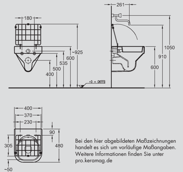
Espital Ausguss , wandhängend, 6 l, mit Edelstahlklapprost, 400 x 480 mm, Modell-Nr. 201680 mit KeraTect®.
