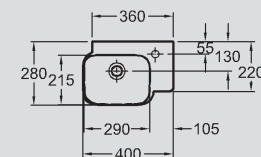
7 Handwaschbecken mit Ablaufkappe Weiß/Chrom, Hahnloch rechts oder links, 400 x 280 mm. Modell-Nr. 125540 rechts. Modell-Nr. 125440 links.
