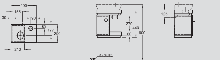
11 Handwaschbecken-Unterschrank, 1 Tür, Türanschlag links, 1 Griff, verchromt, 400 x 440 x 290 mm, Modell-Nr. 816442 Weiß Hochglanz. Kombinierbar mit Handwaschbecken.
