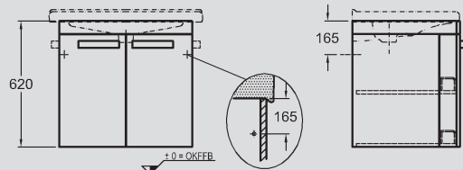
Handtuchhalter, Boden/Zwischenboden optional
