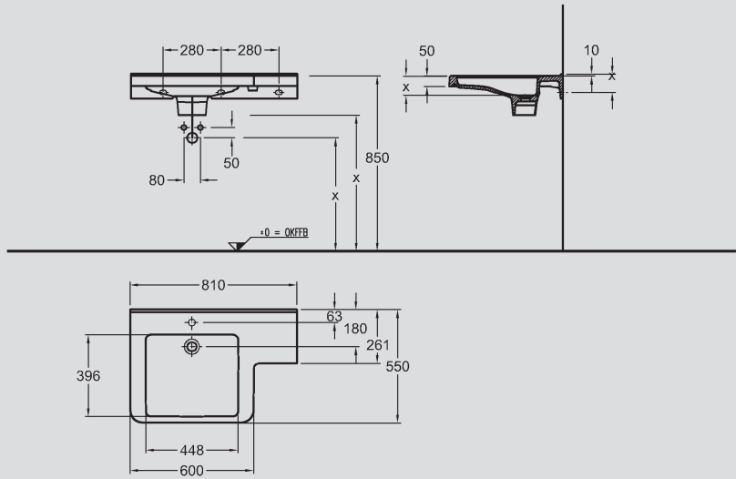
4 Waschtisch aus Varicor®, ohne Überlauf, Ablagefläche rechts, 810 x 550 mm, Modell-Nr. 470085.
