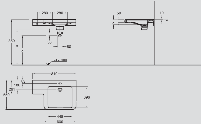
3 Waschtisch aus Varicor®, ohne Überlauf, Ablagefläche links, 810 x 550 mm, Modell-Nr. 470080.
