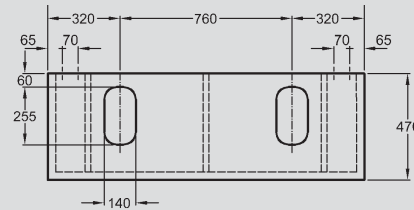
6 Waschtischplatte, Siphonausschnitt links und rechts, umlaufende Blende in Chrom-Optik, inkl. Montagekonsolen, 1400 x 100 x 470 mm, Modell-Nr. 816642 Weiß Hochglanz. Kombinierbar mit 2 Aufsatzwaschtischen, 2 Waschtischen 600 mm, Waschtischunterschrank 600 · 1400 mm, Handtuchhalter 430 · 760 mm und Kosmetik-Modulen.
