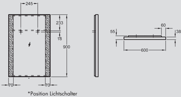
15 Lichtspiegelement, Rahmen verchromt, 2 Leuchten T5 FH, 21 W, 220-240 V, 50-60 Hz, Anti-Beschlag, Lichtschalter, RGB LED's, Fernbedienung, IP 44, Schutzklasse 2, 600 x 900 x 55 mm, Modell-Nr. 816560.
