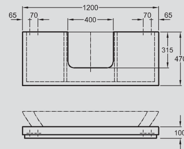
4 Waschtischplatte, Siphonausschnitt mittig, umlaufende Blende in Chrom-Optik, inkl. Montagekonsolen, 1200 x 100 x 470 mm, Modell-Nr. 816620 Weiß Hochglanz. Kombinierbar mit Waschtisch 1000 mm, Waschtisch ohne Hahnlöcher 1200 mm, Waschtischunterschrank 1200 mm, Handtuchhalter 430 mm (seitliche Montage) und Kosmetik-Modulen.
