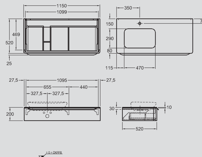
14 Waschtischunterschrank mit Siphonausschnitt links, 1 Auszug, Griff verchromt, 1150 x 200 x 520 mm. Modell-Nr. 814260 Weiß Hochglanz. Modell-Nr. 814261 Taupe Hochglanz. Kombinierbar mit Einbauwaschtisch 600 mm.
