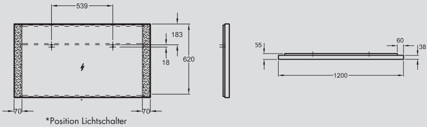
17 Lichtspiegelement, Rahmen verchromt, 2 Leuchten T5 FQ, 24 W, 220-240 V, 50-60 Hz, Anti-Beschlag, Lichtschalter, RGB LED's, Fernbedienung, IP 44, Schutzklasse 2, 1200 x 620 x 55 mm, Modell-Nr. 816520.
