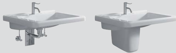
6 Waschtisch, ohne Überlauf, unterfahrbar, DIN 18040, zwei Wasserebenen im Innenbecken, 600 x 550 mm, Modell-Nr. 128662. Kombinierbar mit Halbsäule, Modell-Nr. 298510 oder Waschtischunterschrank 530 mm.
