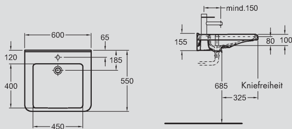
6 Waschtisch, ohne Überlauf, unterfahrbar, DIN 18040, zwei Wasserebenen im Innenbecken, 600 x 550 mm, Modell-Nr. 128662. Kombinierbar mit Halbsäule, Modell-Nr. 298510 oder Waschtischunterschrank 530 mm.
