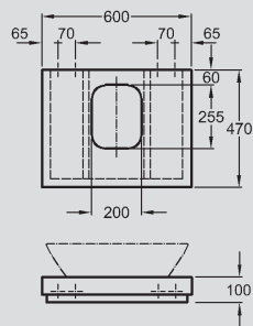
1 Waschtischplatte, Siphonausschnitt mittig, umlaufende Blende in Chrom-Optik, 600 x 100 x 470 mm, Modell-Nr. 816660 Weiß Hochglanz. Einzeln montierbar nur in Verbindung mit Montagekonsolen, Modell-Nr. 516200. Kombinierbar mit Aufsatzwaschtischen, Waschtisch 600 mm, Waschtischunterschrank 600 mm, Handtuchhalter 430 mm (den Montage) und Kosmetik-Modulen.
