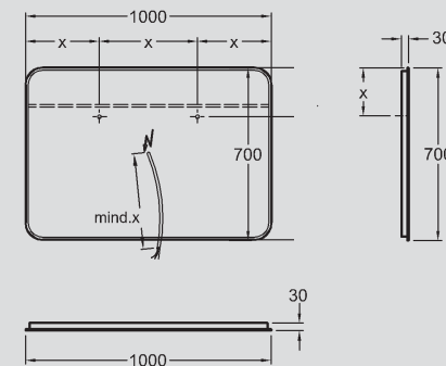
19 Lichtspiegelement, 1000 x 700 x 30 mm, Modell-Nr. 814300.
