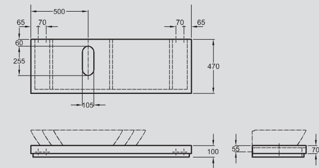
8 Waschtischplatte, Siphonausschnitt links, umlaufende Blende in Chrom-Optik, inkl. Montagekonsolen, 1400 x 100 x 470 mm, Modell-Nr. 816640 Weiß Hochglanz. Kombinierbar mit Aufsatzwaschtisch, Ablagefläche links, Waschtischen 600 · 800 · 1000 mm, Waschtischunterschrank 600 · 1400 mm, Handtuchhalter 430 · 760 mm und Kosmetik-Modulen.
