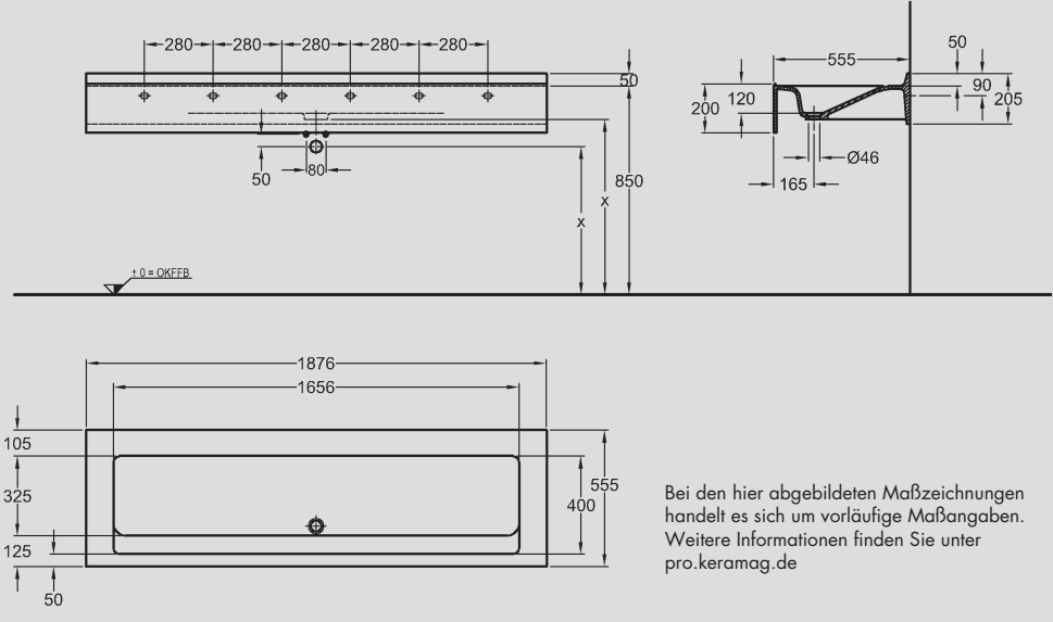
Active Waschrinne aus Varicor®, 1876 x 205 x 555 mm. Modell-Nr. 401876016 Weiß (Alpin). Modell-Nr. 401876095 Duocolor-Weiß.
