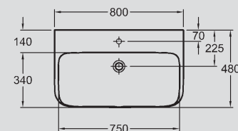
3 Waschtisch mit Ablaufkappe Weiß/Chrom, 800 x 480 mm, Modell-Nr. 125480. Kombinierbar mit Halbsäule, Modell-Nr. 291410 und Waschtischunterschränken 680 mm. Auch mit Ab- und Überlaufsystem Clou erhältlich.
