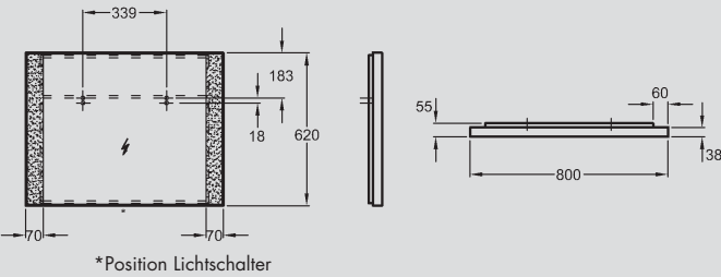
16 Lichtspiegelement, Rahmen verchromt, 2 Leuchten T5 FQ, 24 W, 220-240 V, 50-60 Hz, Anti-Beschlag, Lichtschalter, RGB LED's, Fernbedienung, IP 44, Schutzklasse 2, 800 x 620 x 55 mm, Modell-Nr. 816580.
