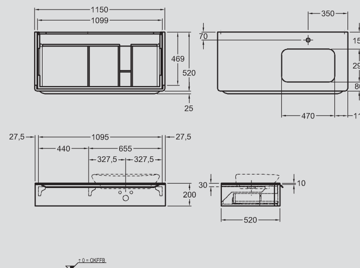
13 Waschtischunterschrank mit Siphonausschnitt rechts, 1 Auszug, Griff verchromt, 1150 x 200 x 520 mm. Modell-Nr. 814160 Weiß Hochglanz. Modell-Nr. 814161 Taupe Hochglanz. Kombinierbar mit Einbauwaschtisch 600 mm.
