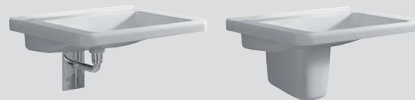
7 Waschtisch, ohne Hahnloch, ohne Überlauf, unterfahrbar, DIN 18040, zwei Wasserebenen im Innenbecken, 600 x 550 mm, Modell-Nr. 128661. Kombinierbar mit Halbsäule, Modell-Nr. 298510 oder Waschtischunterschrank 530 mm.
