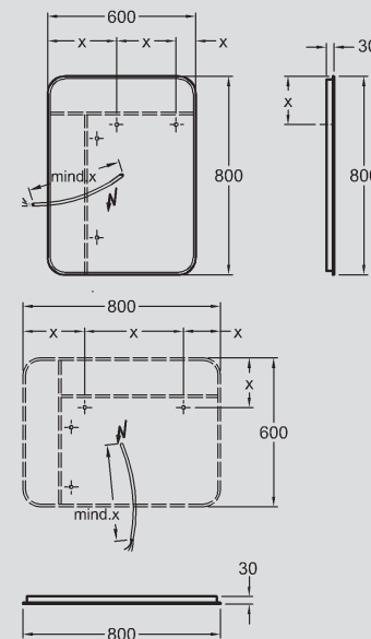
18 Lichtspiegelement, 600 x 800 x 30 mm, Modell-Nr. 814360.
